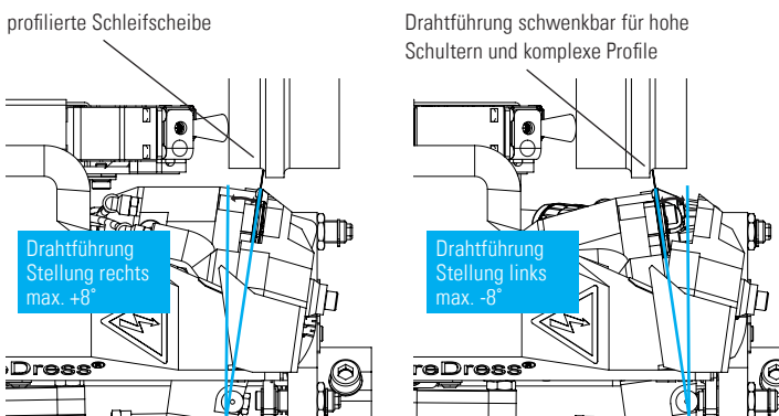
Grafik Schwenkbarkeit, mit Beispiel Scheibenprofil
