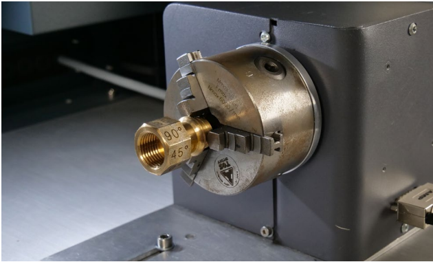
Gravieren von zylindrischen Teilen
