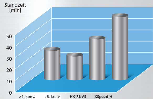
Standzeit HDC-Fräsen in 1.2379
